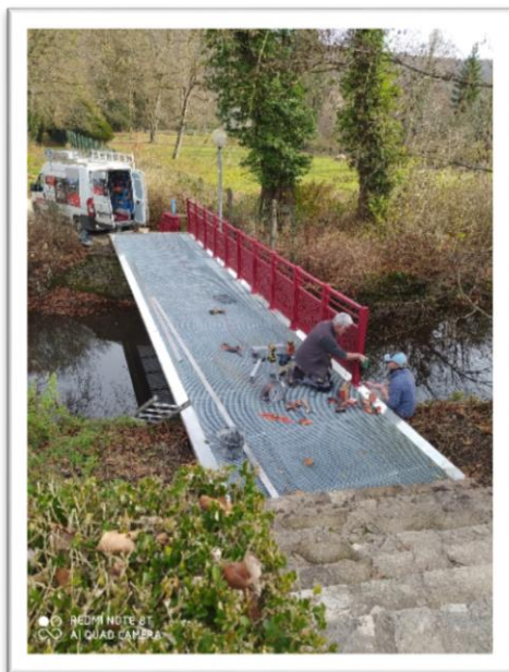
POSE DES GARDE-CORPS
